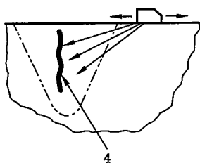
b) 厚度方向上的典型示例
