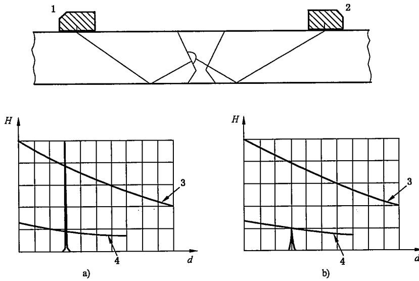
图 B.1 检测方向示例
