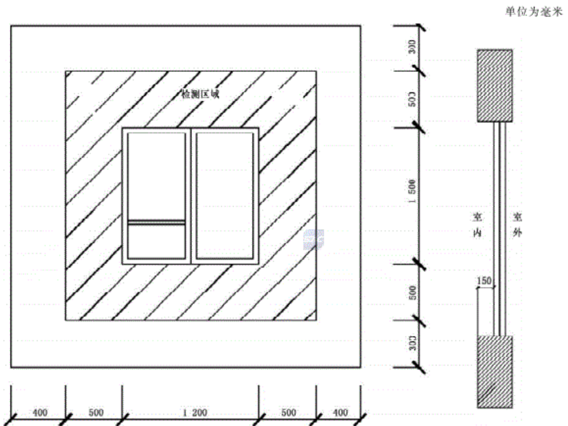
图 A.1 外窗洞口区域正视图与剖断面示意图
