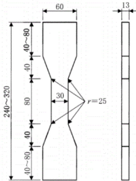
图1 拉伸性能用试件
