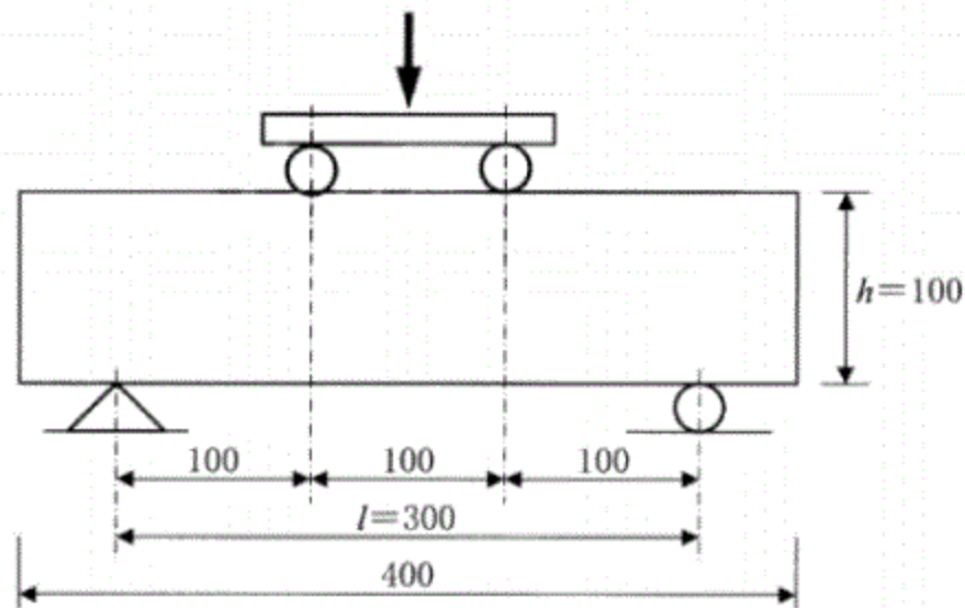
图3 抗折强度试验装置
