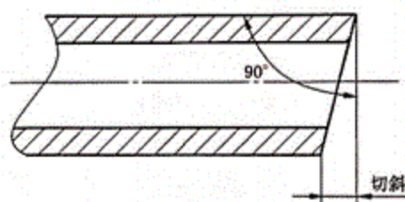
图 1 切斜
