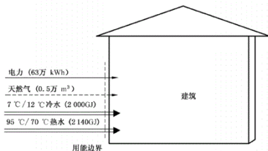
图 C.1 建筑能耗示例
