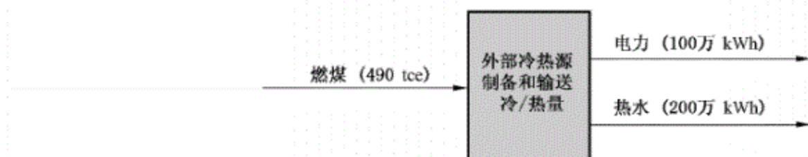
图 C.3 建筑所需热水的制备和输送系统及能耗案例 2
