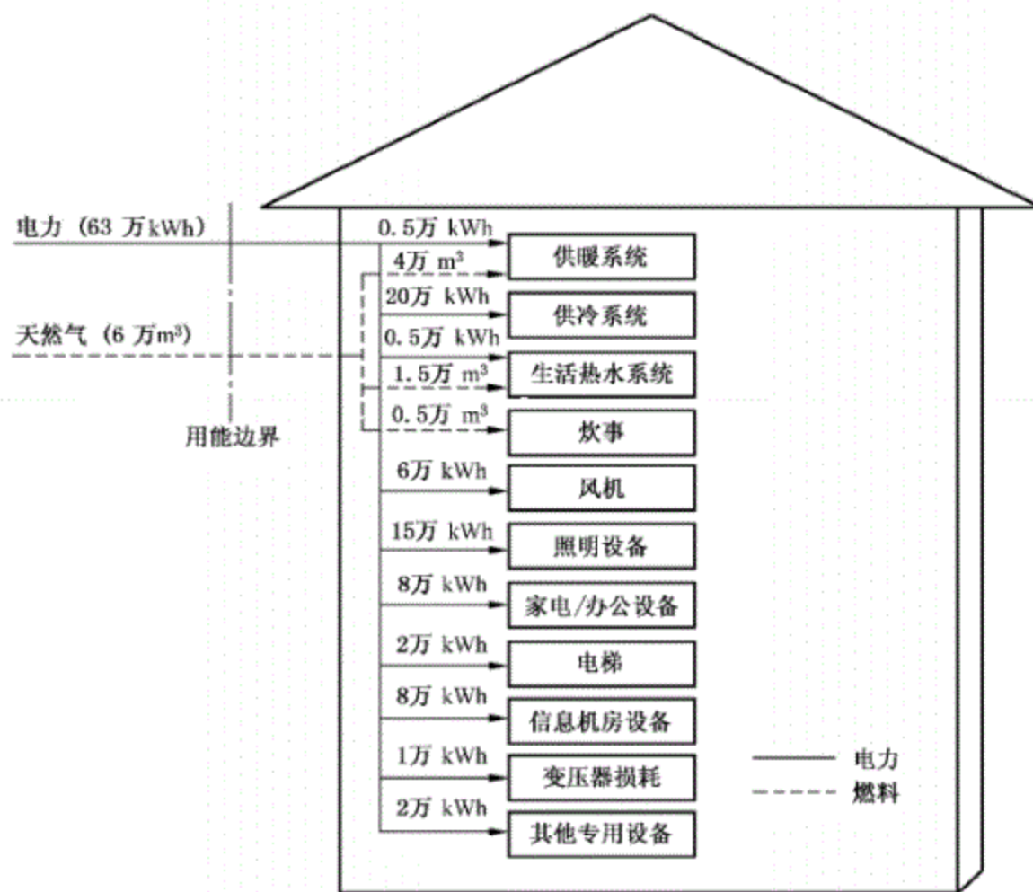
图 A.1 建筑能耗表述示例
