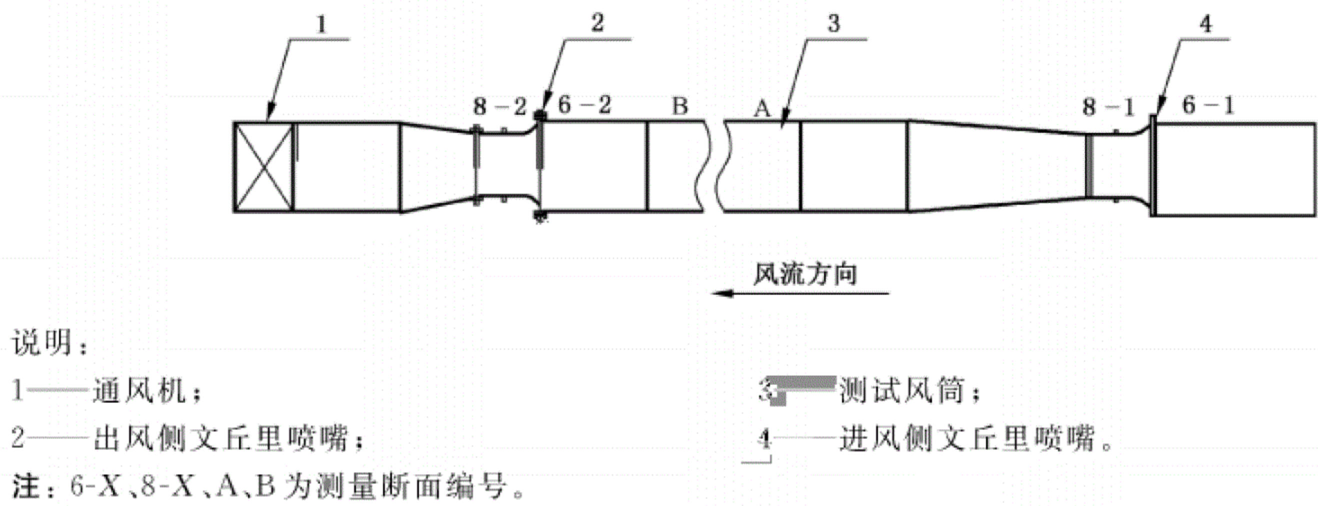
图 2 负压风筒测量装置示意图(单文丘里喷嘴时)
