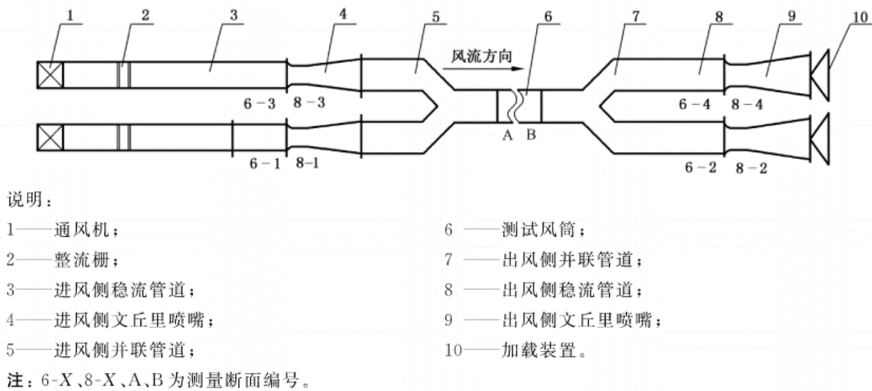
图 1 正压风筒测量装置示意图(文丘里喷嘴并联时)
