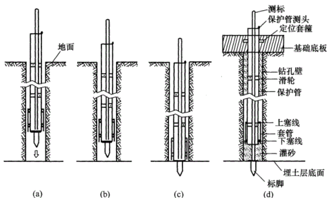
图 25 钻孔法埋设分层沉降标志
