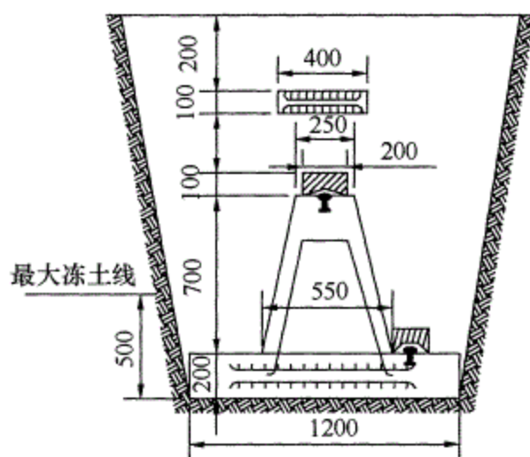
图 14 混凝土基本水准标石 (单位: mm)
