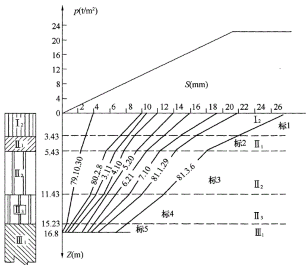
图 26 各土层荷载-沉降-深度曲线
