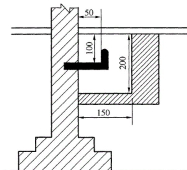
图 32 窰井式标志 (适用于建筑内部埋设，单位：mm)
