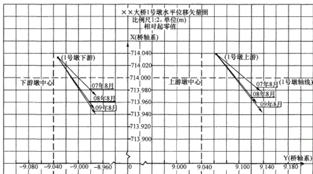
图 37 水平位移图
