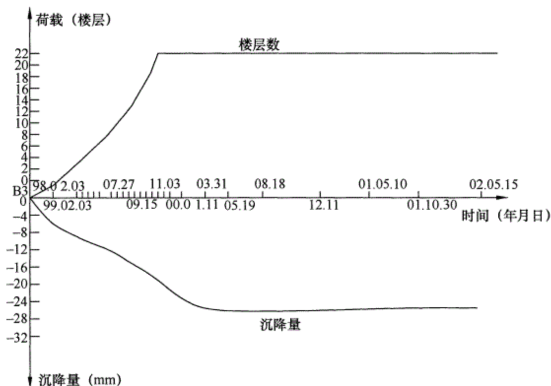
图 35 时间-荷载-沉降量曲线
