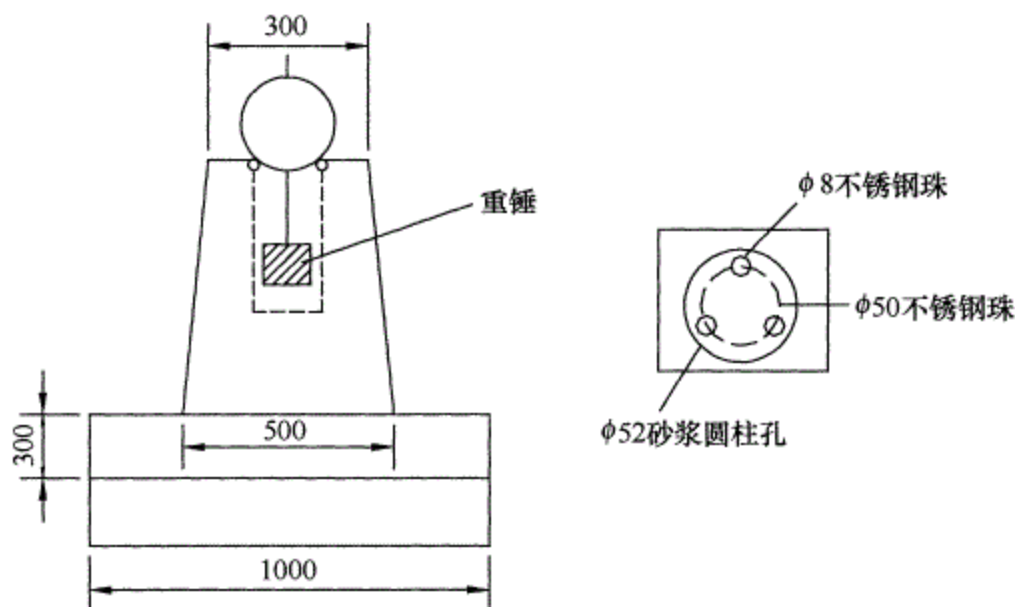
图 21 重力平衡球式照准标志 (单位: mm)
