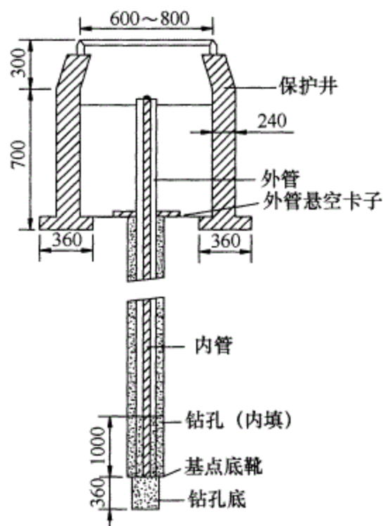
图 13 深埋钢管水准基点标石 (单位: mm)
