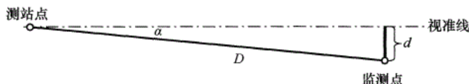
图 4.5.6 小角法示意图
