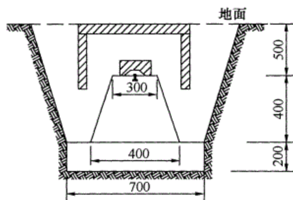
图 15 浅埋钢管水准标石
