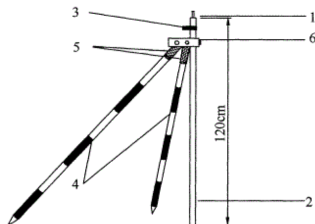
图5 架设棱镜组的三脚架
