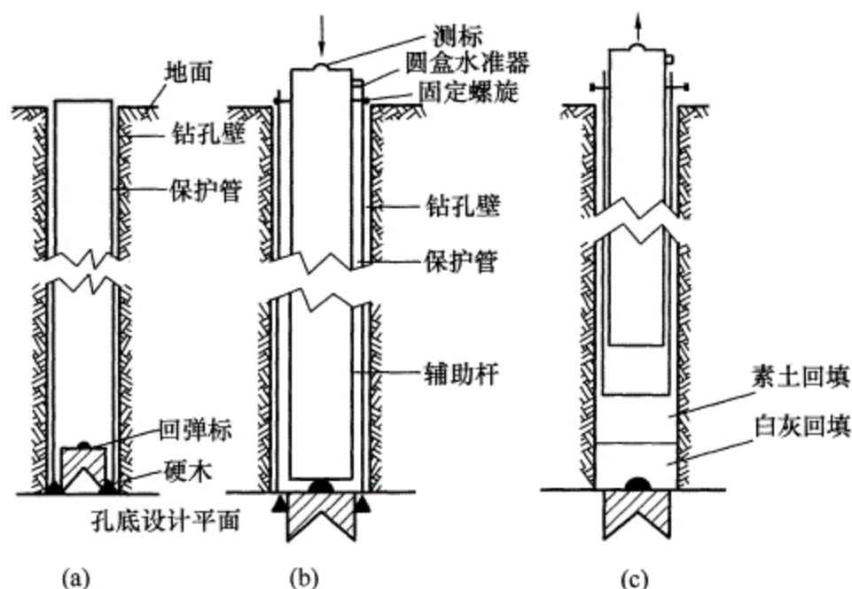
图 29 辅助杆压入式标志埋设步骤
