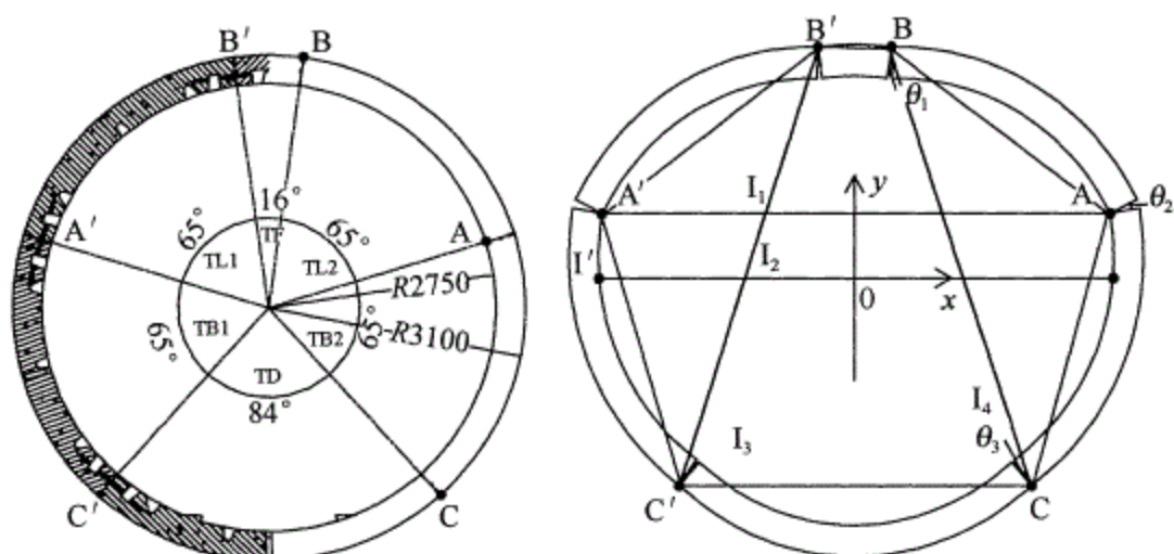
图 39 典型的收敛变形示意图
