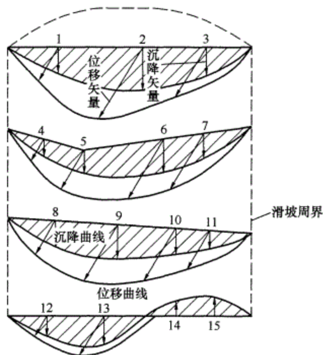
图 28 某斜坡监测点位移综合曲线图
