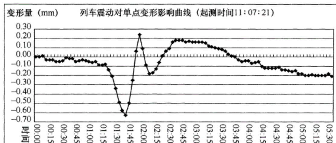
图 3 静力水准典型液面振荡曲线
