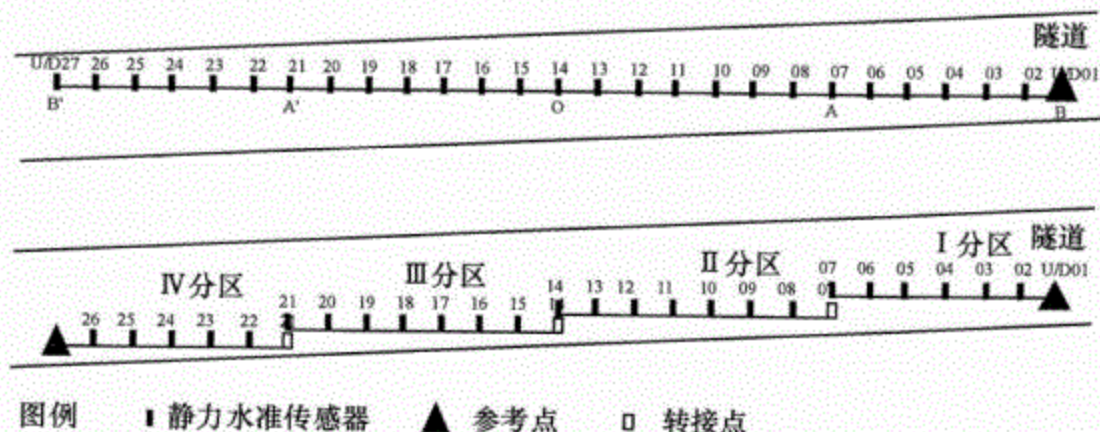
图2 静力水准线路分组安装示意图
