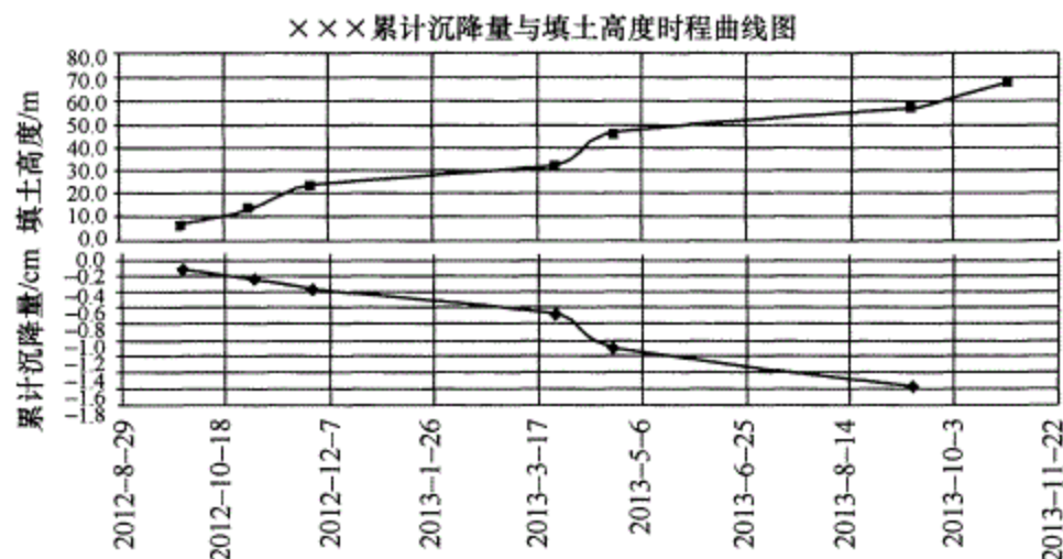
图 27 各土层沉降量-填土高度时程曲线
