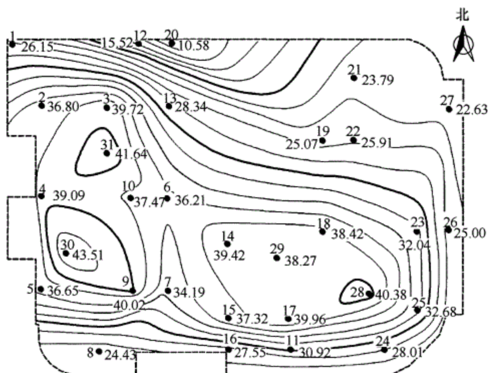
图 36 等沉降曲线
