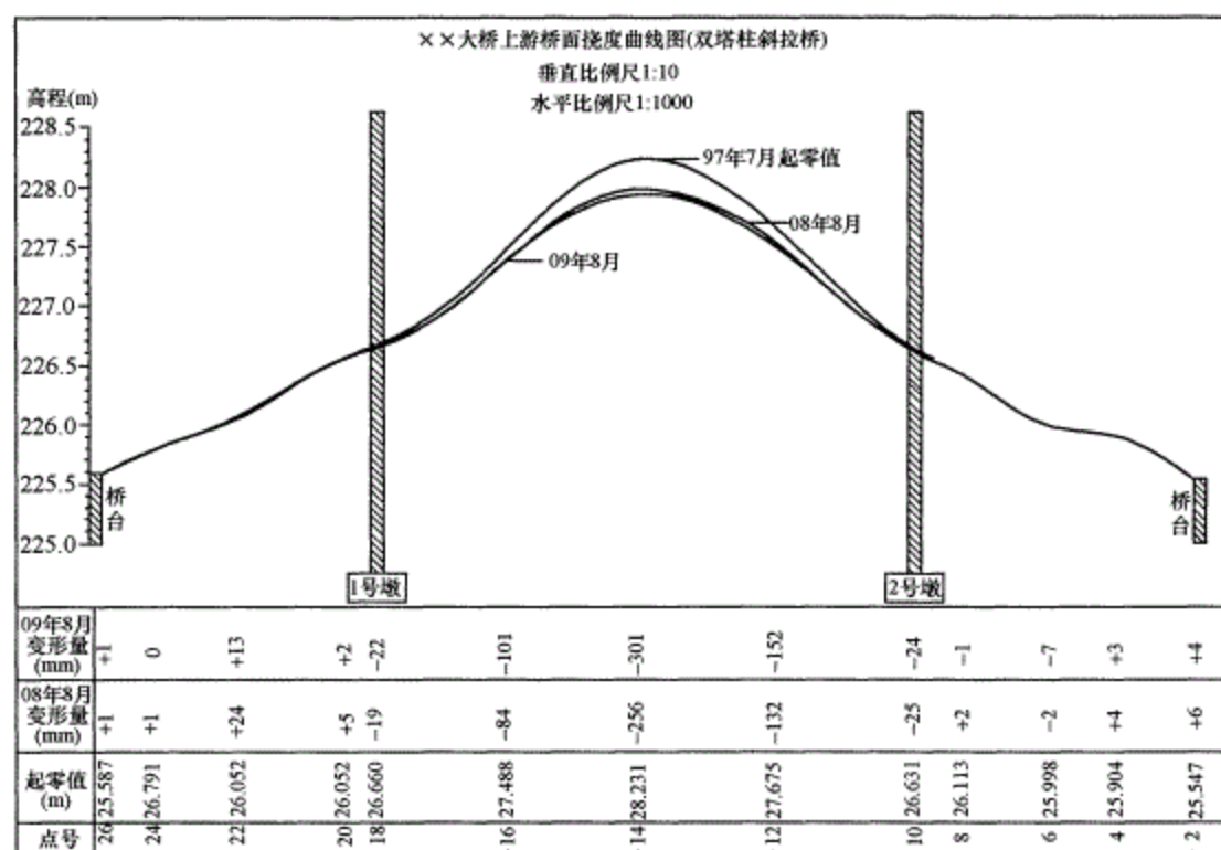
图 38 挠度曲线
