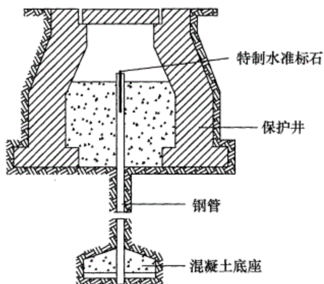
图 15 浅埋钢管水准标石
