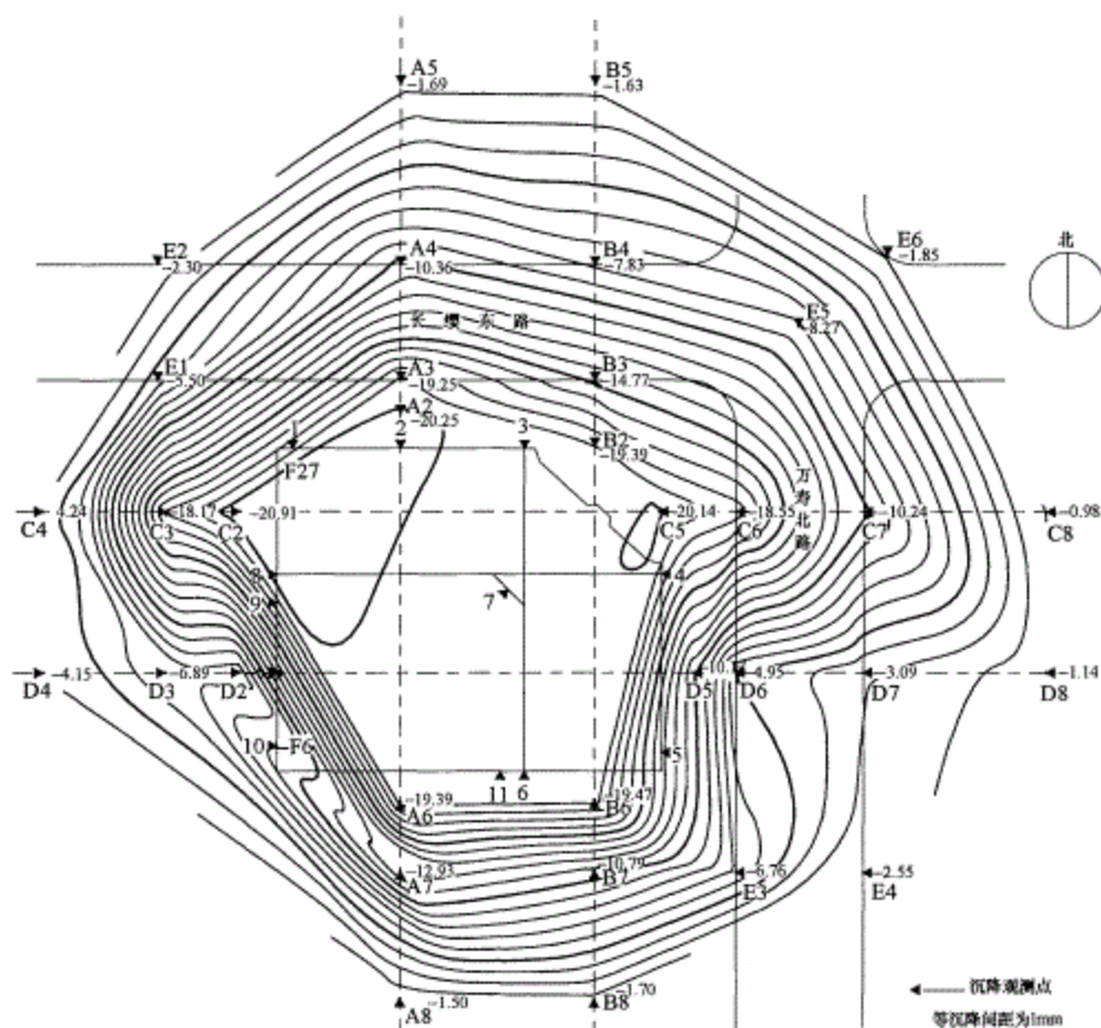
图23 场地地面等沉降曲线
