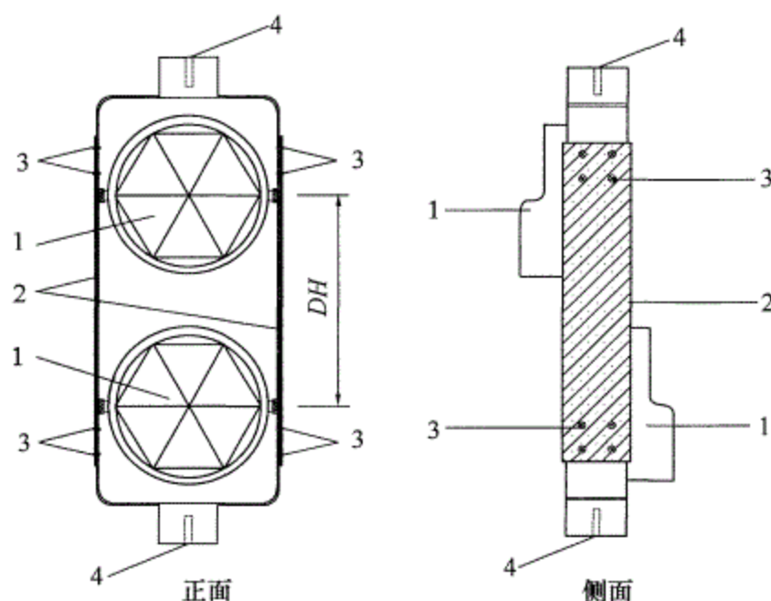
图 4 精密三角高程测量高低棱镜组
