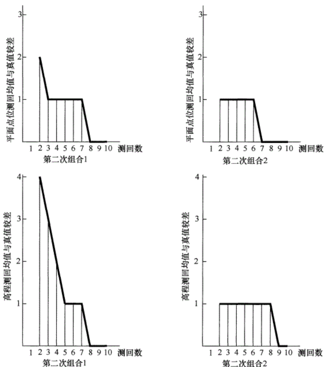
图 9 变换测站后的激光扫描测量平面位置及高程与测回数关系
