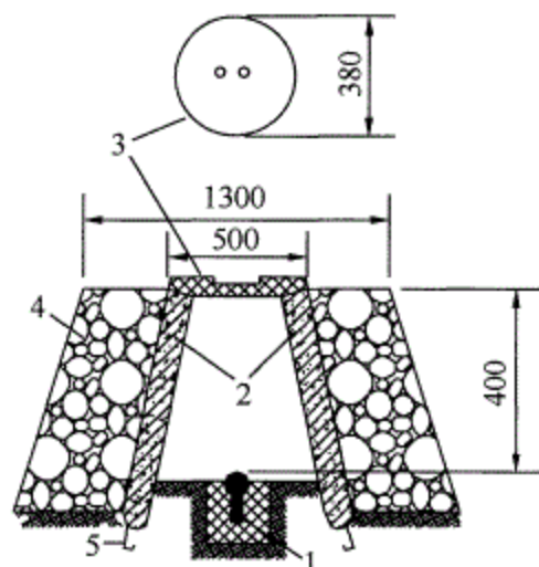
图 11 基岩水准基点标石 (单位: mm)
