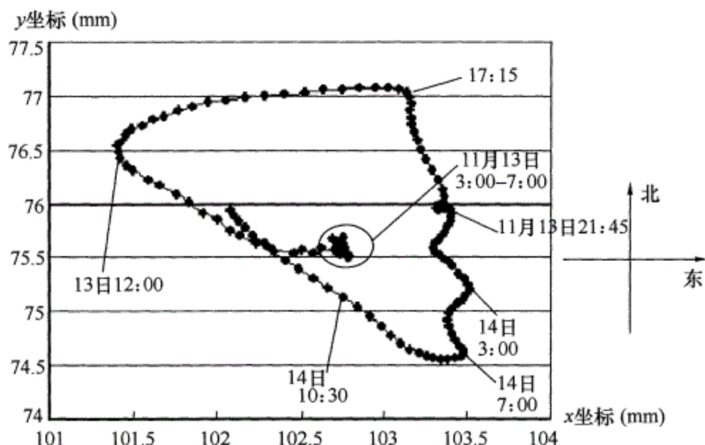
图 42 某超高层建筑日照变形曲线
