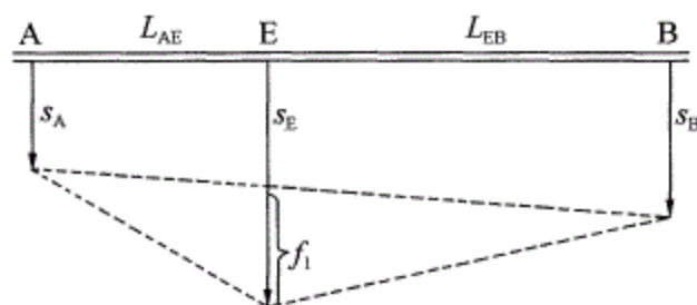
图 7.5.3 竖向的挠度
