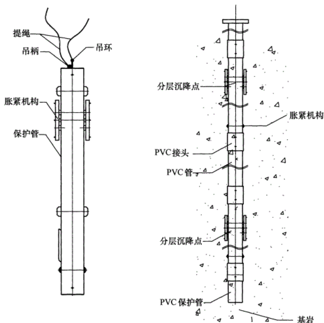
图 24 钻孔法埋设分层沉降计
