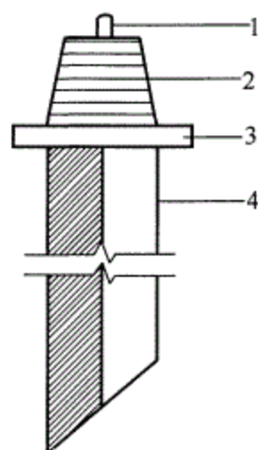
图 30 钻杆送入式标志
