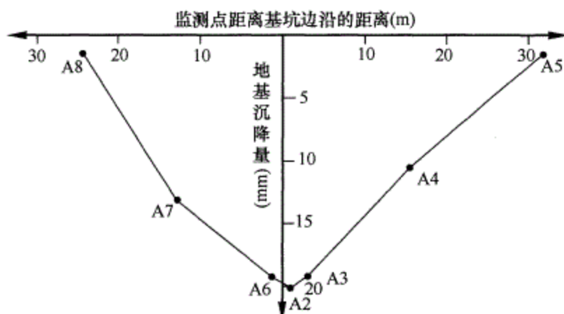
图22 相邻地基沉降的距离-沉降曲线
