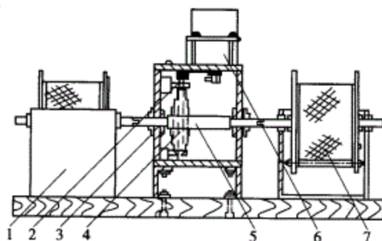
图 T0207-1 耐崩解性试验仪
