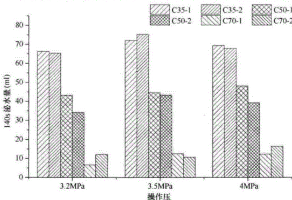
图 5 操作压对不同工作性混凝土拌合物 140s 泌水量的影响
