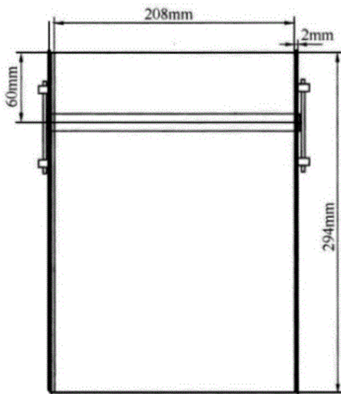
图 17.0.2 盛料器形状和尺寸
