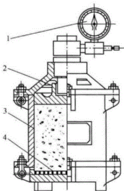
图 13.0.3 压力泌水仪
