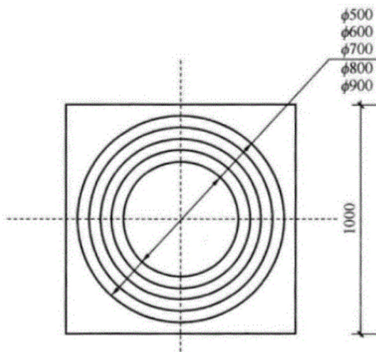
图 10.0.2 底板 (mm)
