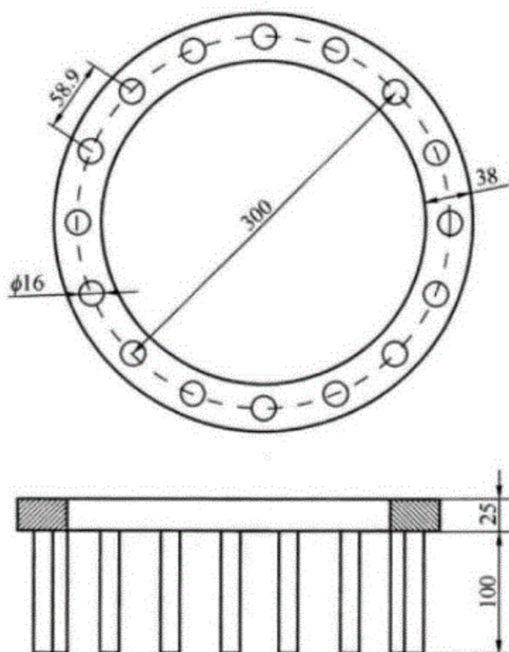
图 8.0.2 J 环示意图 (mm)
