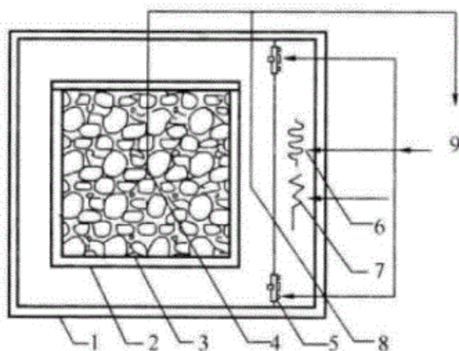
图 19.0.2 绝热温升试验装置
