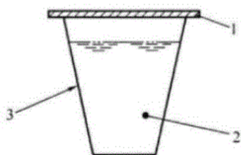
图 7 BS EN 12350-11: 2010 试样容器及盖子
