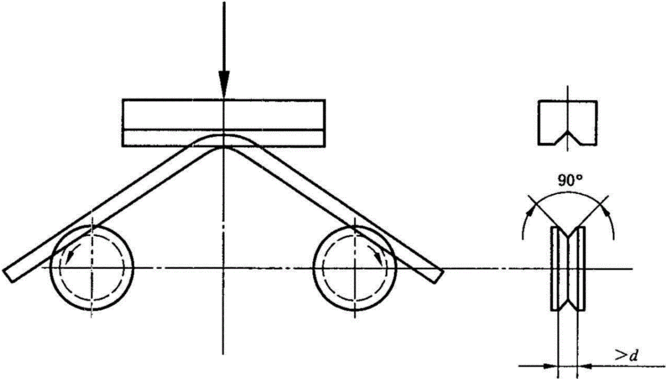
图3 反向弯曲装置的图例
