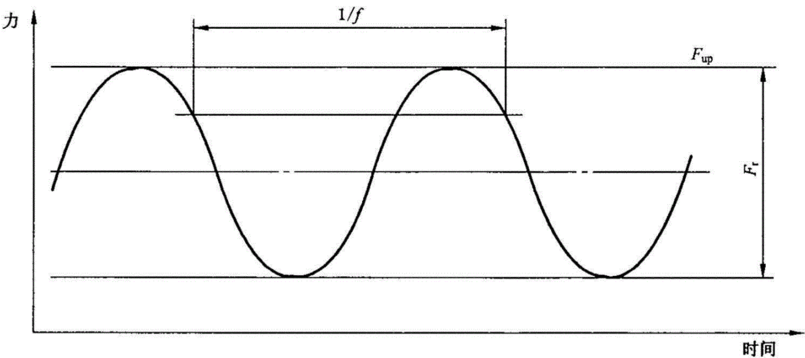
图 5 疲劳加载循环图
