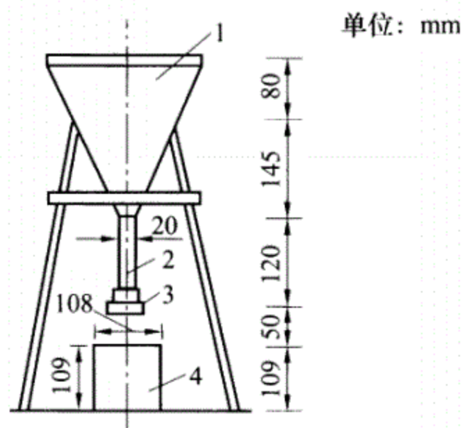
图 3.9.2 漏斗示意图
