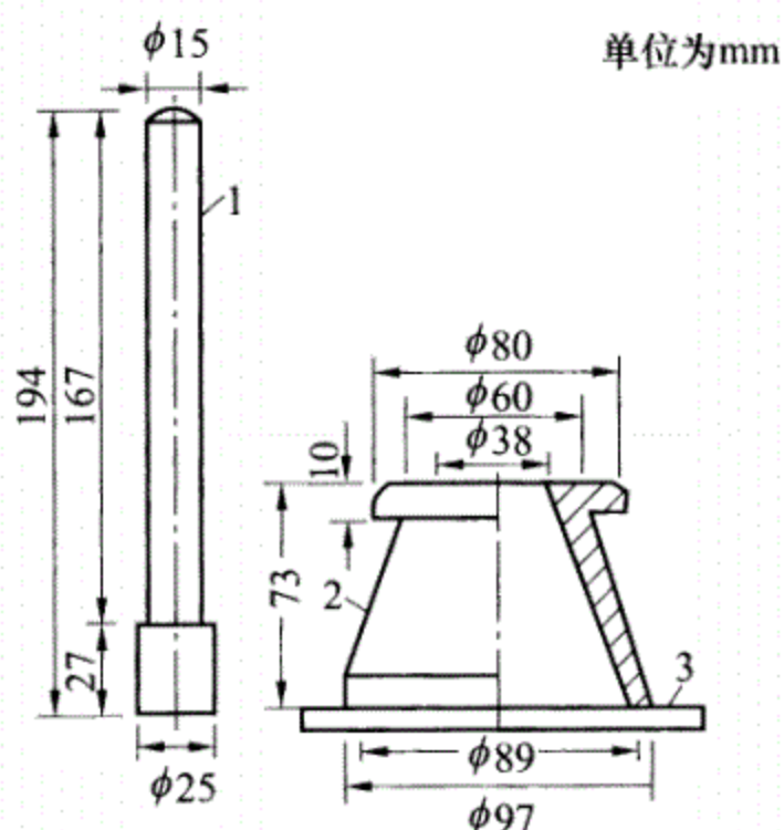
图 3.2.2 饱和面干试模与捣棒
