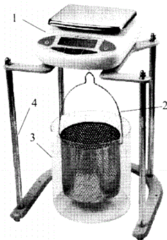
图 4.2.2 水中称量装置示意图
