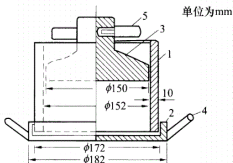
图 4.11.2 压碎指标测定试模
