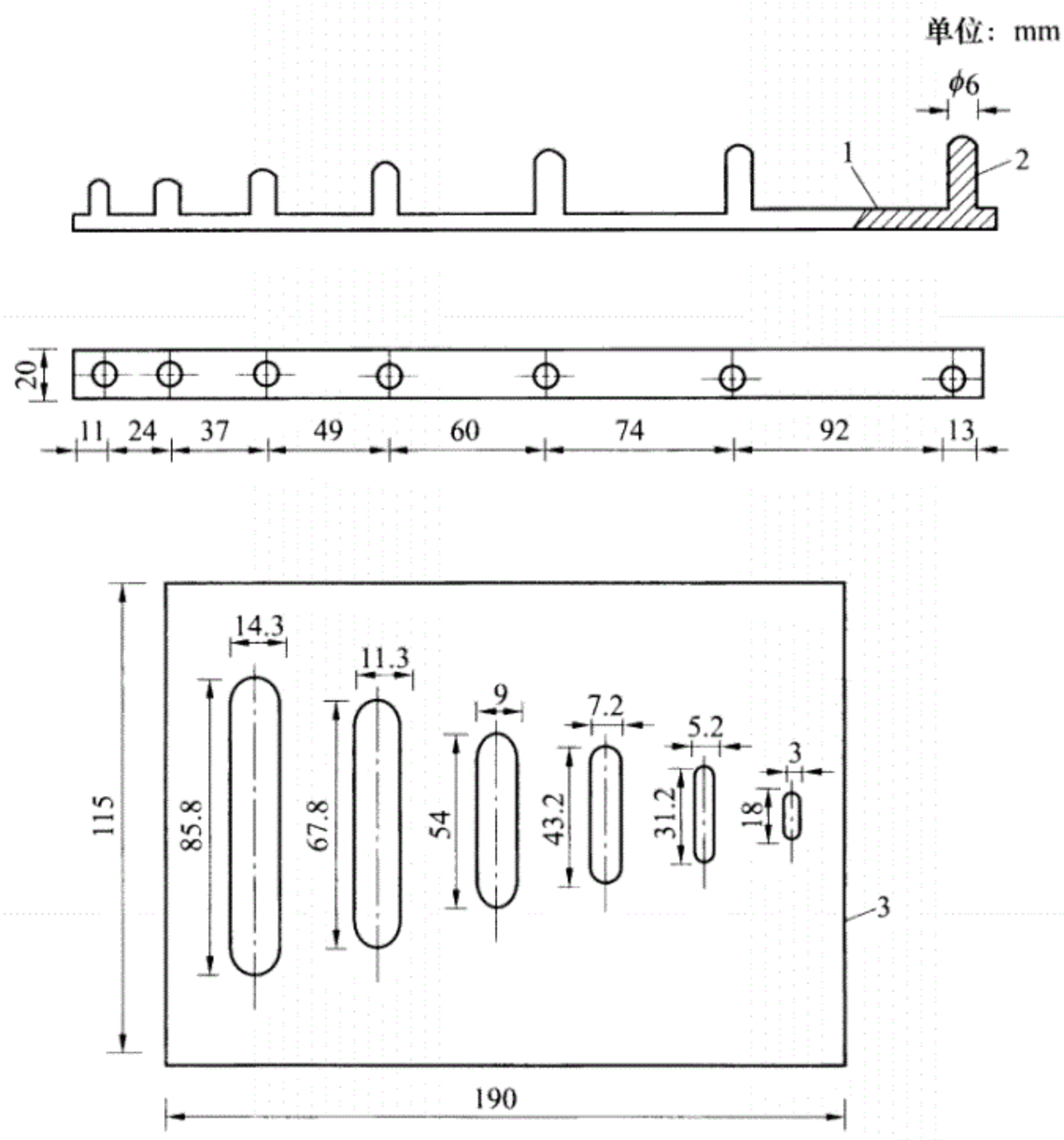
图 4.8.2 针、片状规准仪
