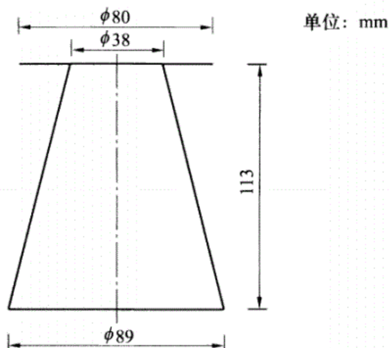
图 3.4.2 人工砂饱和面干试模
