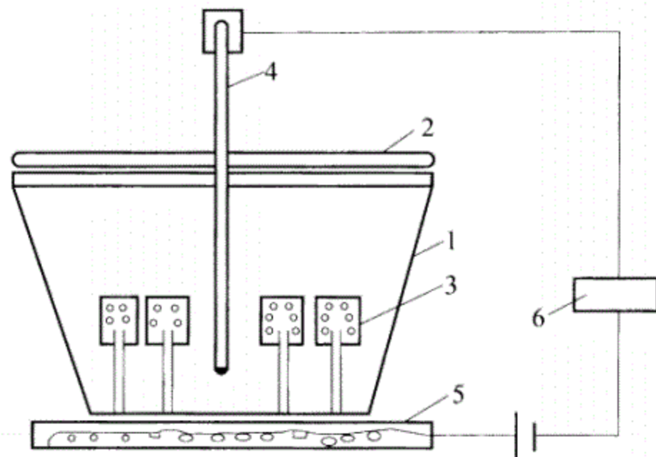
图 3.18.2 恒温试验箱示意图
