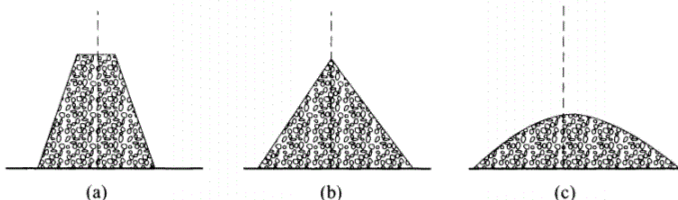
图 3.2.4 饱和面干试验试样形状
