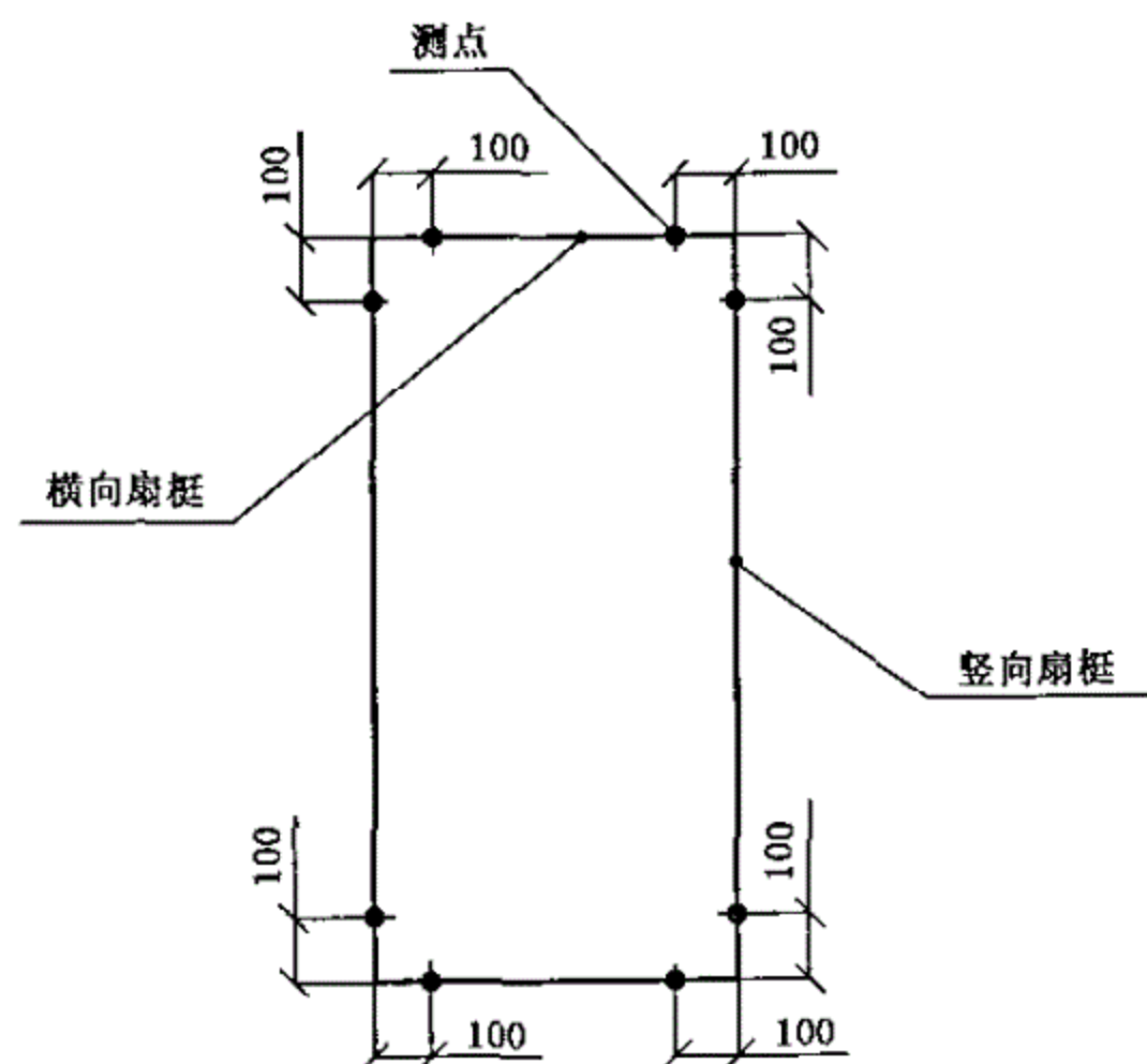
图 1 门窗扇与框的相对位置测点示意
